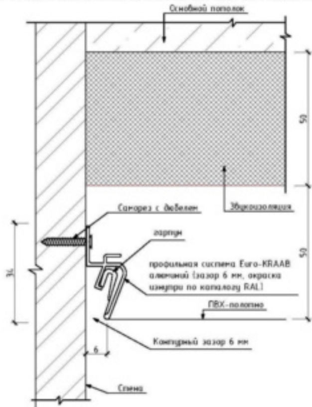
1-1. КОНТУРНАЯ СИСТЕМА КРЕПЛЕНИЯ ПОТОЛКА ПВХ EUROKRAAB
